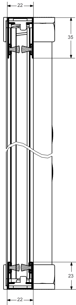
SEZ. VERTICALE
