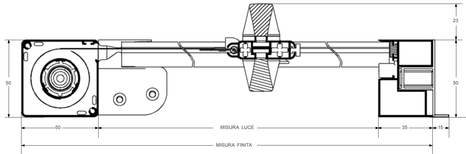
SEZ. ORIZZONTALE
