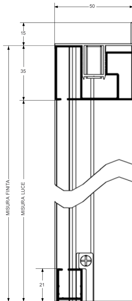
SEZ. VERTICALE
