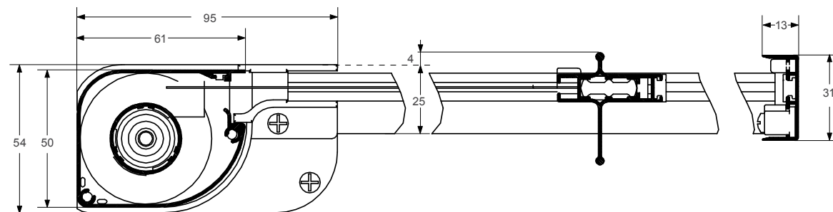
SEZ. ORIZZONTALE
